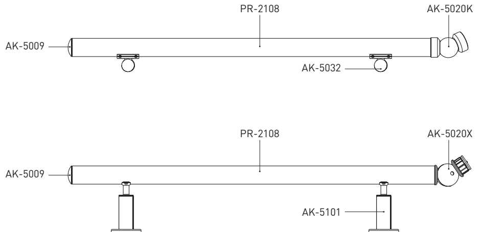
AK-5163 For 400 Handrail 400 Kûpeste uyumlu
